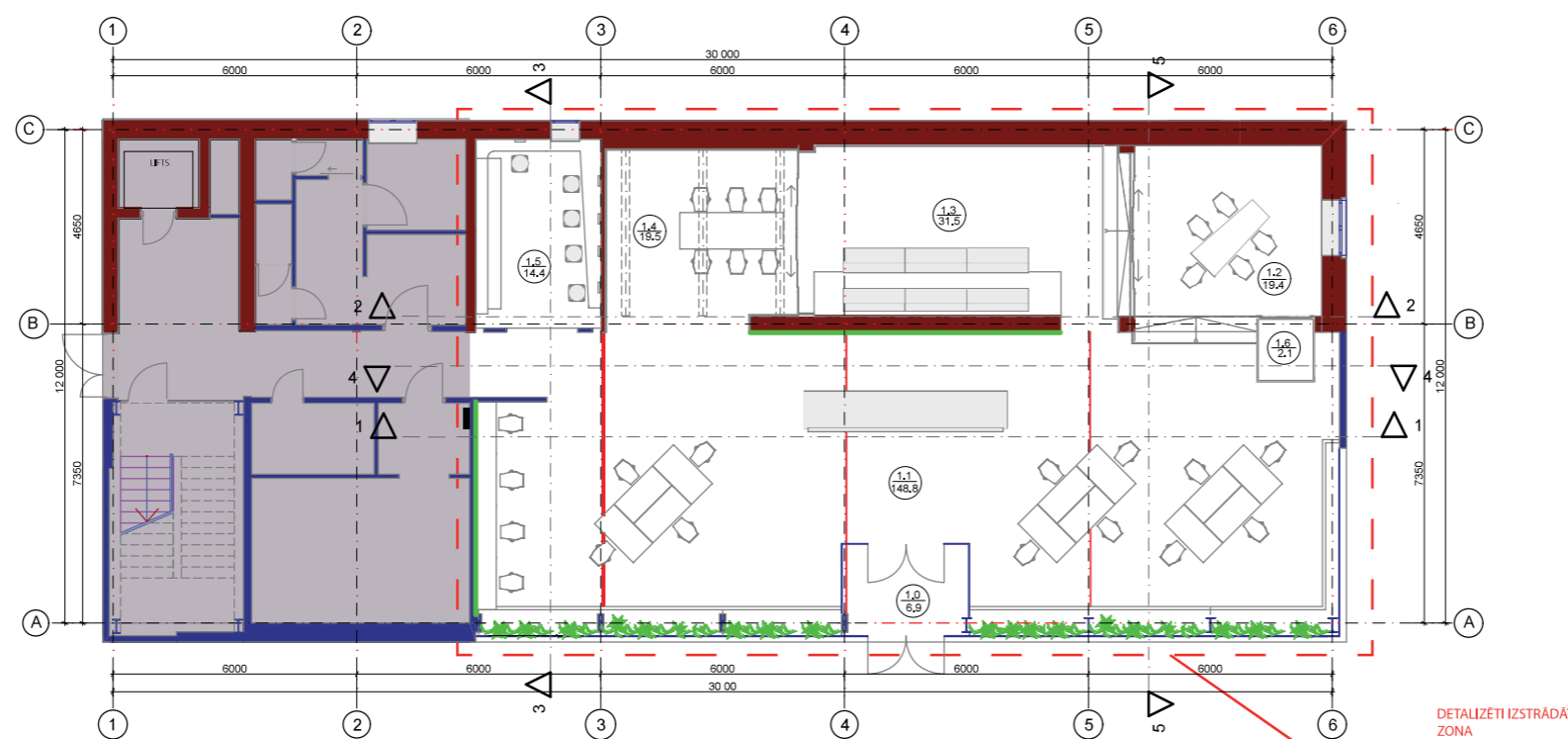
1. stāva plāns, kas ir 3D modeļa griezumus 1m augstumā no stāva grīdas līmeņa, rasējums jau ar pēcapstrādi
